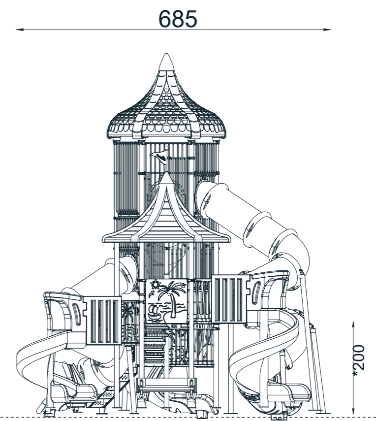
YAN GÖRÜNÜŞ / SIDE VIEW
