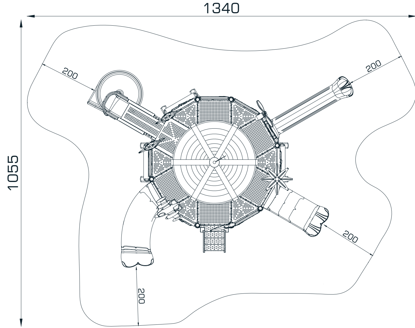
ÜST GÖRÜNÜŞ / TOP VIEW
