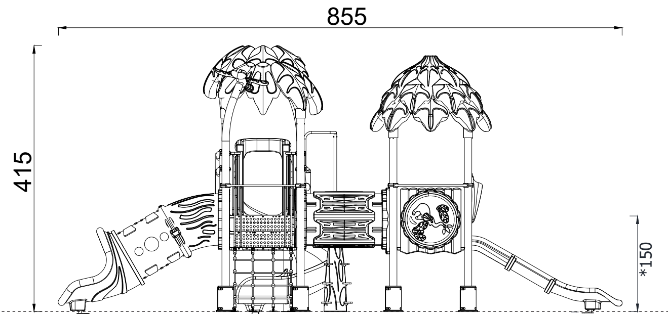
YAN GÖRÜNÜŞ / SIDE VIEW
