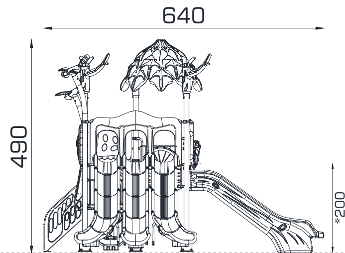
ÖN GÖRÜNÜŞ / FRONT VIEW
