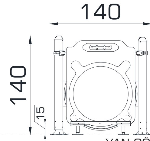
YAN GÖRÜNÜŞ / SIDE VIEW
